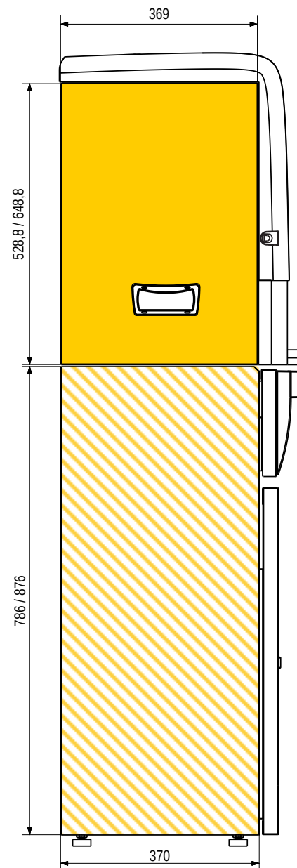
fianco sinistro left side
